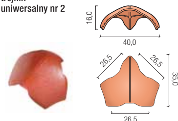
trójkąt uniwersalny nr 2
