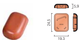
czapa kominka odpowietrzającego
