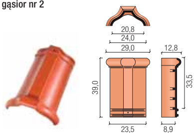
gąsior nr 2
