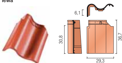
szczytowa lewa
