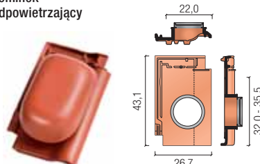
czapa kominka odpowietrzającego
