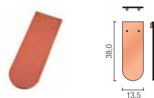
dachówka 5/4
