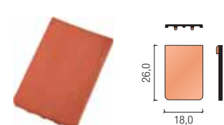
okapowa wentylacyjna
