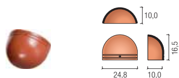
zamknięcie początkowe kalenicy nr 11
