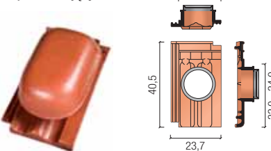
kominek odpowietrzający
