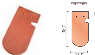
wykrojona went. lewa - "łuska"
