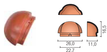
zamknięcie początkowe grzbiotu
