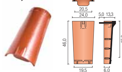
gąsior końcowy kalenicy nr 20
