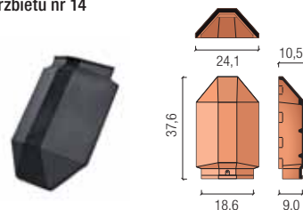
gąsior nr 14
