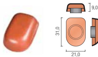
antenowa + nasadka
