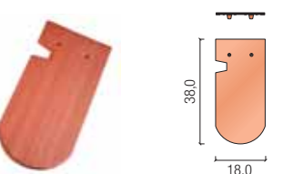
wykrojona went. lewa - "koronka"
