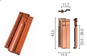
półówkowa
