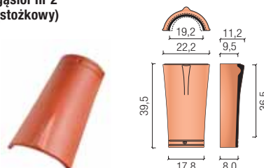
gąsior nr 2 (stożkowy)
