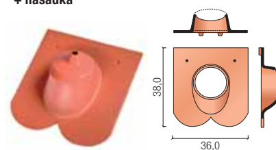
kominek odpowietrzający
