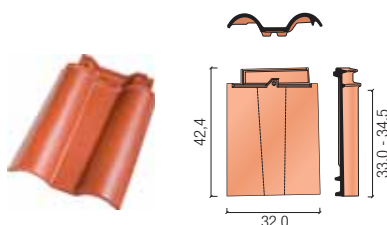
wentylacyjna
