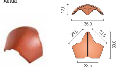
trójkąt uniwersalny Actua
