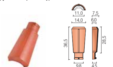
gąsior nr 5 (wieżowy)
