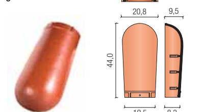
gąsior początkowy grzbietu nr 20
