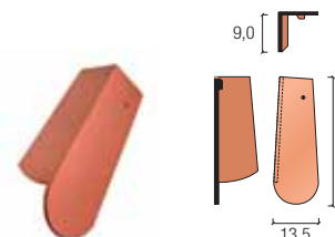
szczytowa 3/4 prawa
