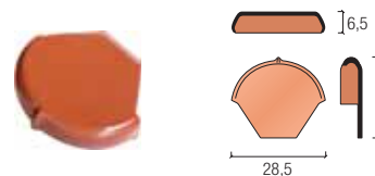
zamknięcie końcowe kalenicy nr 11
