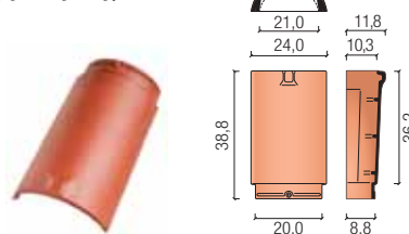
gąsior nr 2 (stożkowy)
