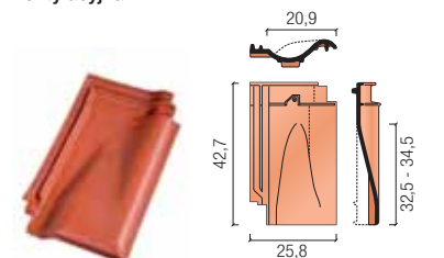
wentylacyjna
