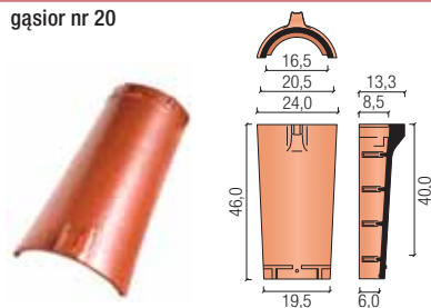
gąsior początkowy kalenicy nr 20
