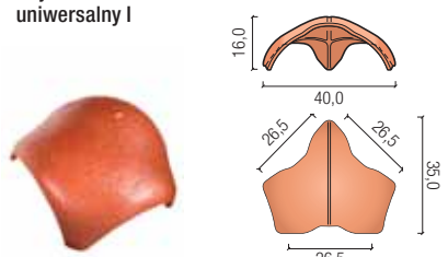
trójkąt uniwersalny I
