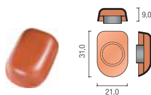
czapa kominka odpowietrzającego
