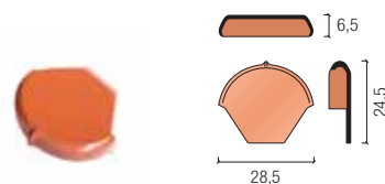
trójkąt początkowy nr 11
