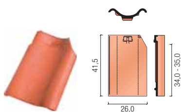
dwufalowa
