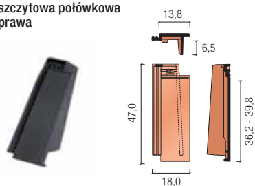
połówkowa
