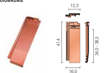
zamykająca lewa
