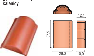
zamknięcie początkowe grzbiotu
