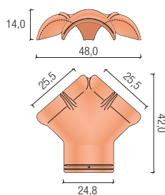
trójkąt początkowy nr 11
