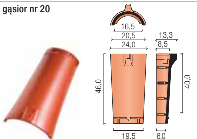
gąsior nr 20
