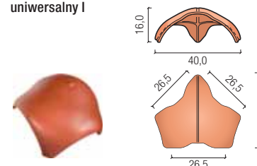
trójkąt uniwersalny I
