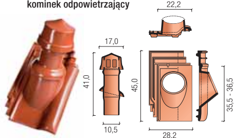
kominek odpowietrzający
