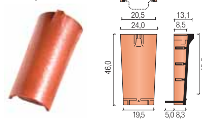
gąsior początkowy grzbietu nr 20
