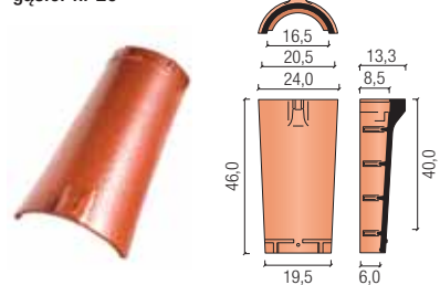
gąsior początkowy kalenicy nr 20
