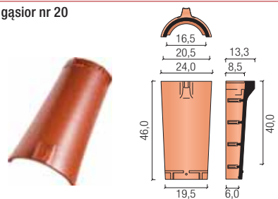
gąsior nr 20
