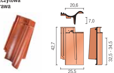
dwufalowa
