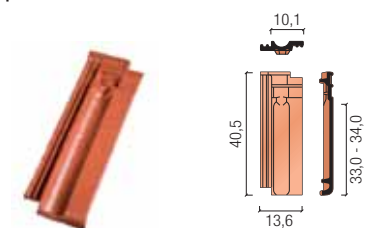
połówkowa
