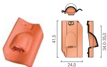
dwufalowa
