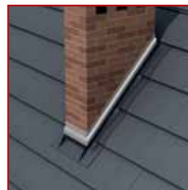
Taśma i profil do obróbki komina
