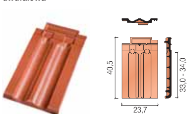
dwufalowa
