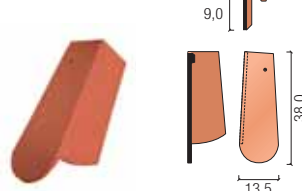
szczytowa 3/4 prawa
