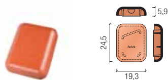
czapa kominka odpowietrzającego
