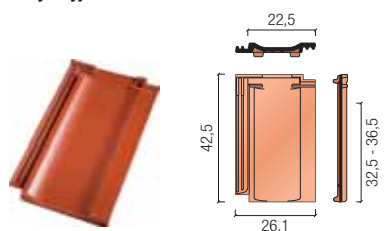
wentylacyjna
