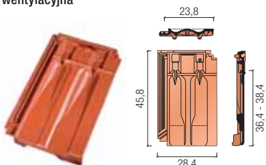
wentylacyjna
