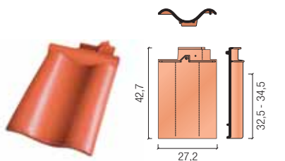
wentylacyjna
