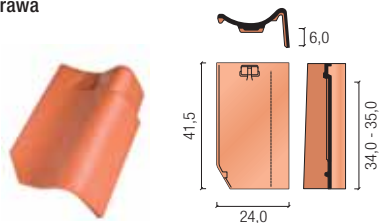
wentylacyjna
