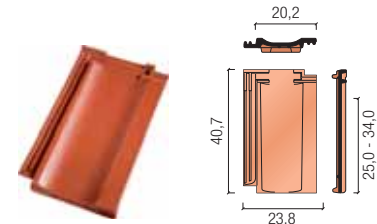
wentylacyjna
