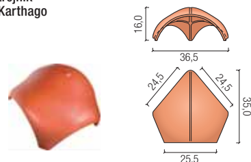
trójkąt Karthago
