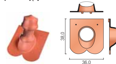
kominek odpowietrzający
