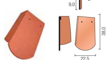
szczytowa 5/4 lewa
