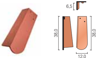
szczytowa 1/2 prawa
