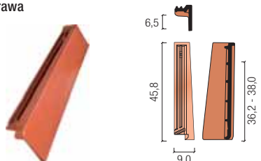
wentylacyjna
