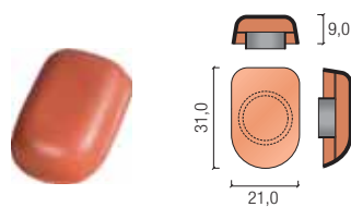
antenowa + nasadka
