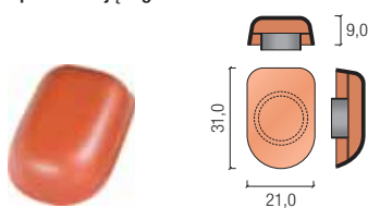
czapa kominka odpowietrzającego
