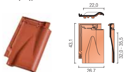
wentylacyjna
