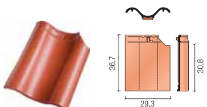
dwufalowa
