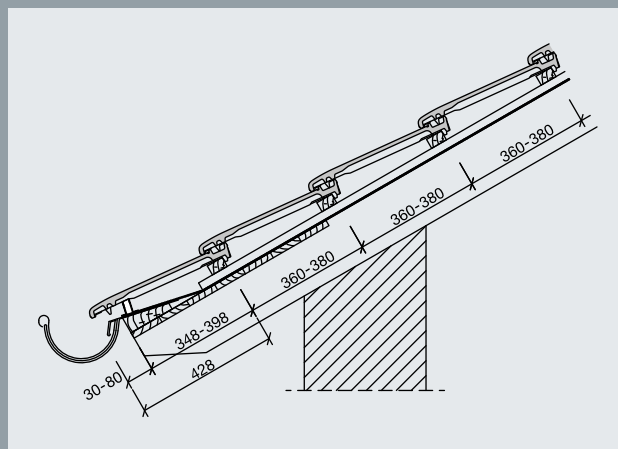
UKŁAD KALENIC Z GĄSIOREM PLANO
