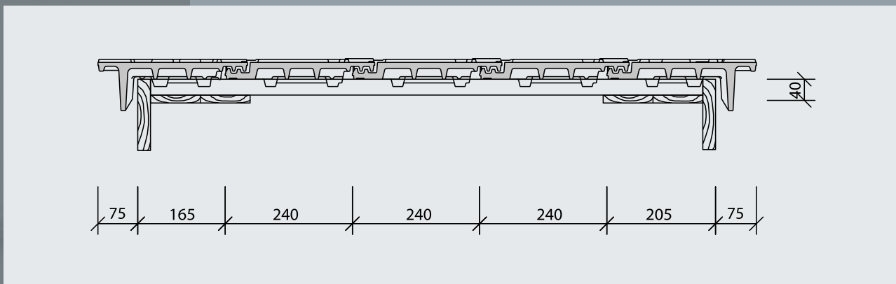
UKŁAD DACHÓWEK SZCZYTOWYCH PLANO
