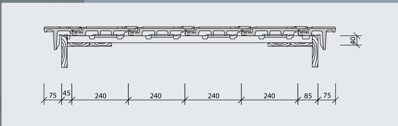
UKŁAD DACHÓWEK SZCZYTOWYCH PLANO 1/2
